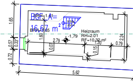
Keller
