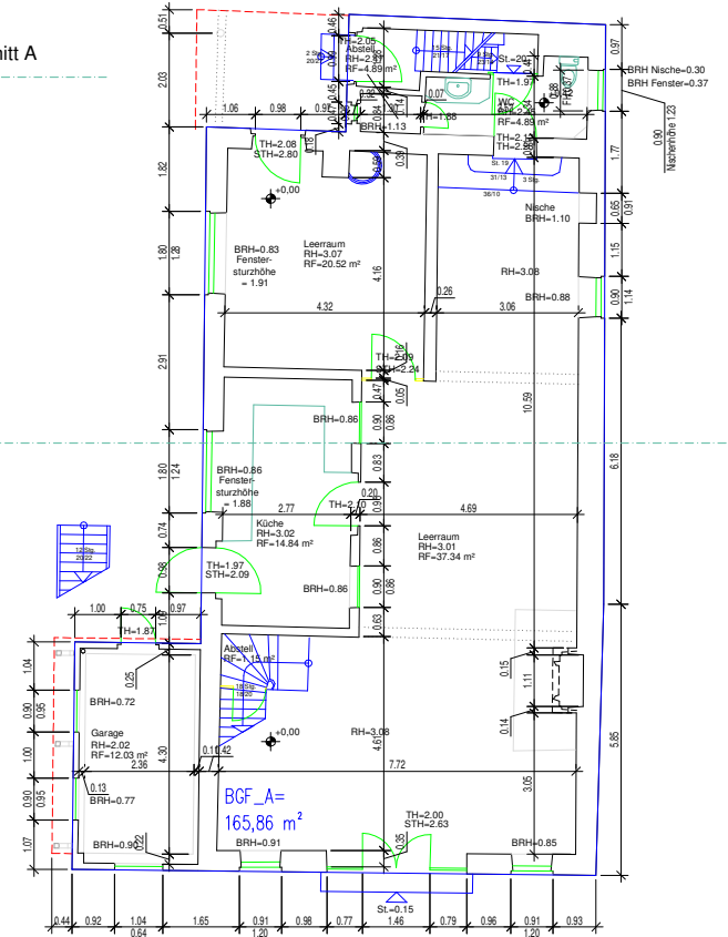
Erdgeschoss
